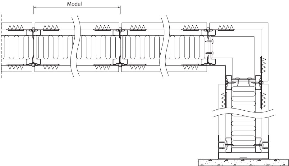
Vandret snit
