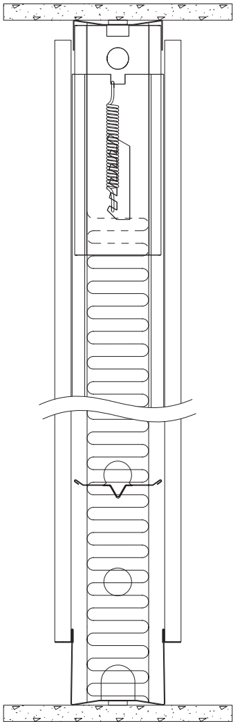
Lodret snit
