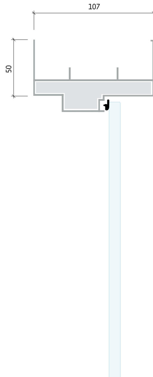
Glasdør i 2 lags glasvæg
