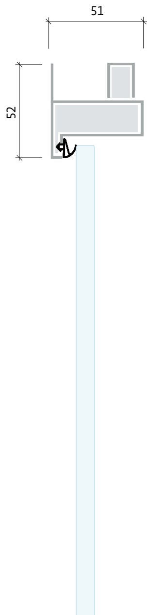
Glasdør i T-karm (Vægtype R_w 34 - 42 dB)
