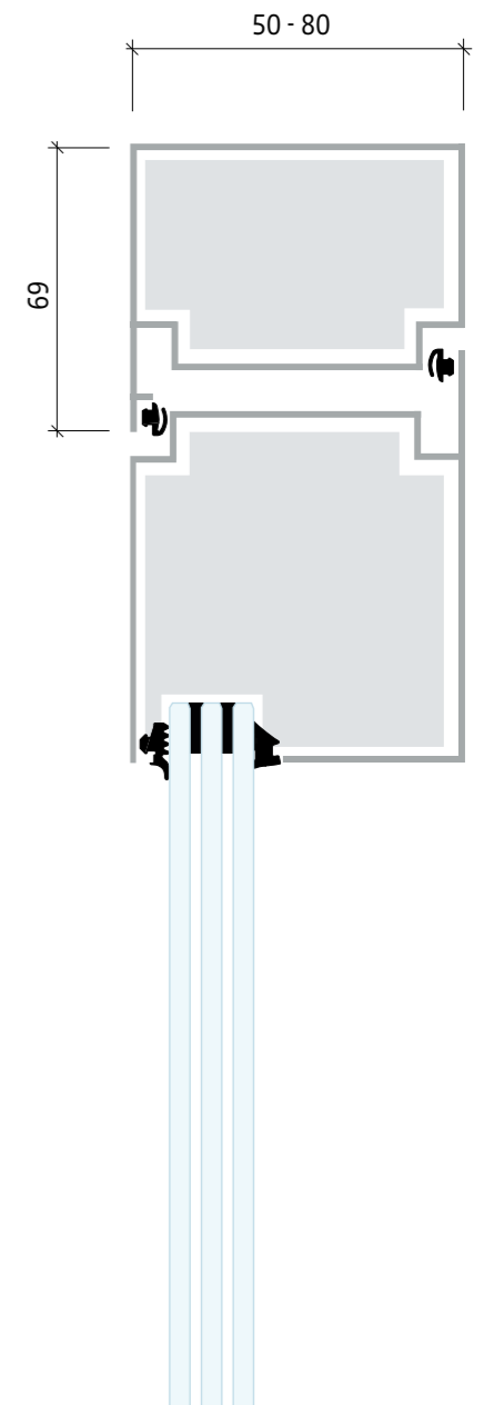
Alu-rammeglasdør
