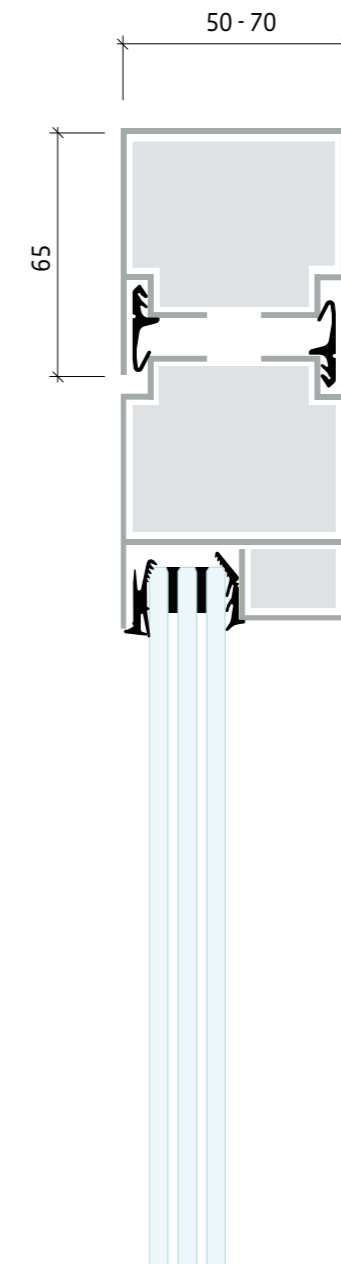
Stålramme-glasdør
