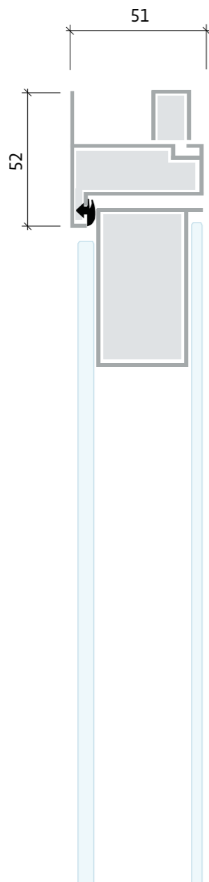
Glasrammedør i T-karm
